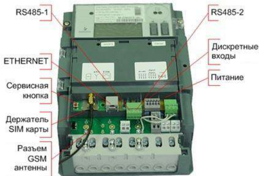
Рисунок 4.6 Элементы подключения модуля телемеханики
