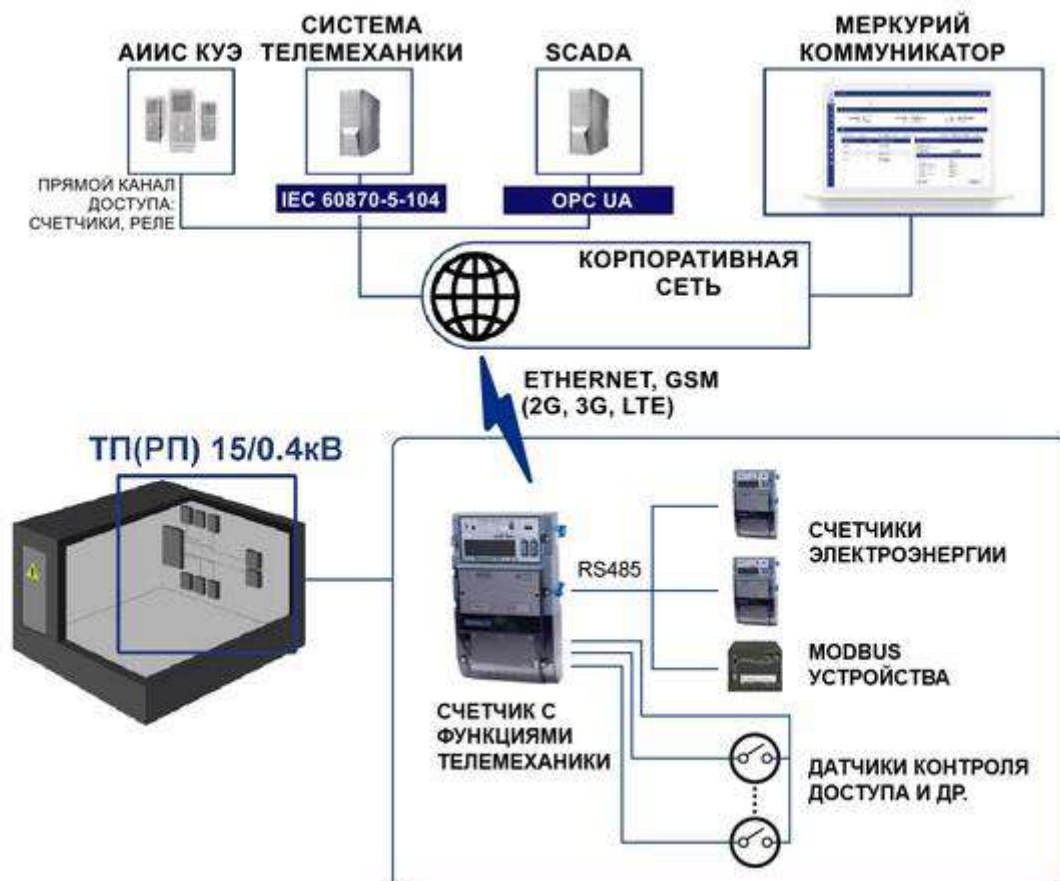
Рисунок 3.4 – Схема работы в составе автоматизированных систем
