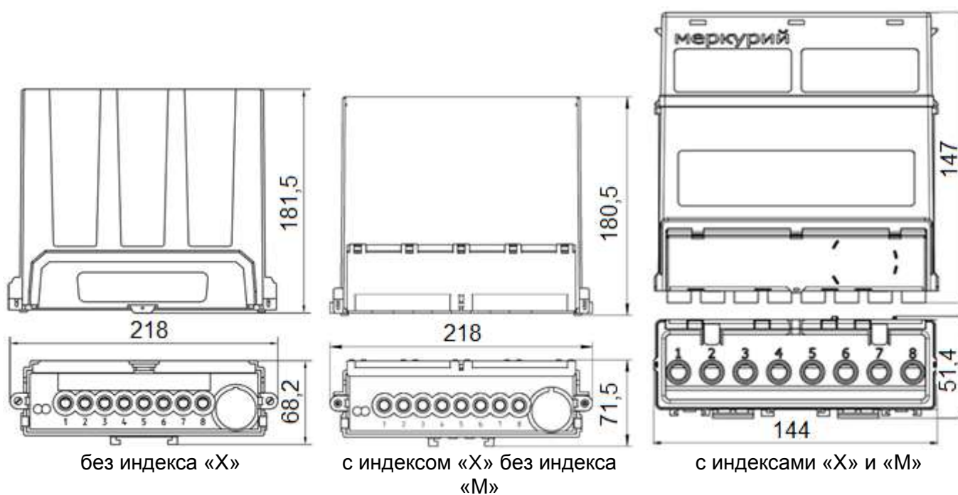
Рисунок А.4 – Габаритные чертежи модификаций счетчика «Меркурий 238»
